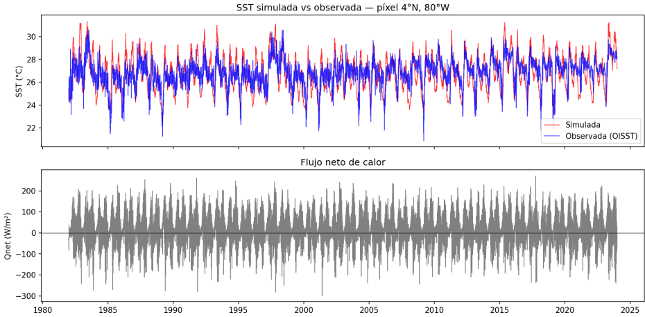
Figura 2: Validación temporal del modelo PWP en el píxel de referencia (4°N, 80°W), 1982–2023. Panel superior: SST simulada (rojo) y SST observada OISST v2.1 (azul). Panel inferior: flujo neto de calor en superficie ( Q_{\text{net}} ) calculado por el modelo.
